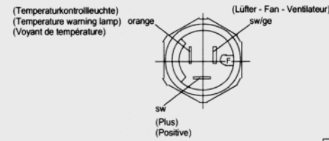
Kabelanschluss Thermoschalter (Draufsicht) Thermostat cable connection (top view) Câble de connexion, thermocontact (vue en plan)
